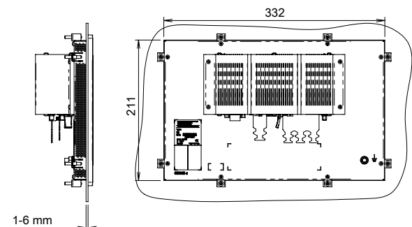
Montage / Einbauausschnitt Assembly / Installation cut-out
